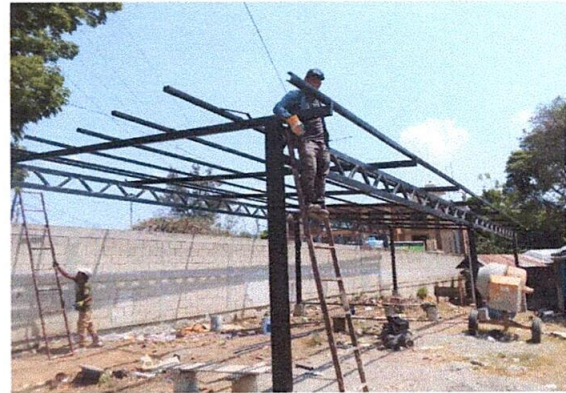
Foto 2: Estructura de techo.
